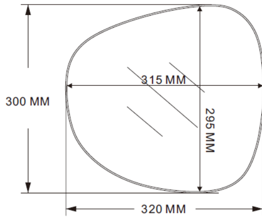
正面图
