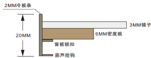
剖面图
